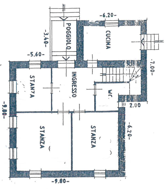
PIANO TERRA h. = 3.25
