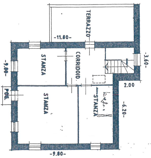
PIANO PRIMO h. = 3.25
