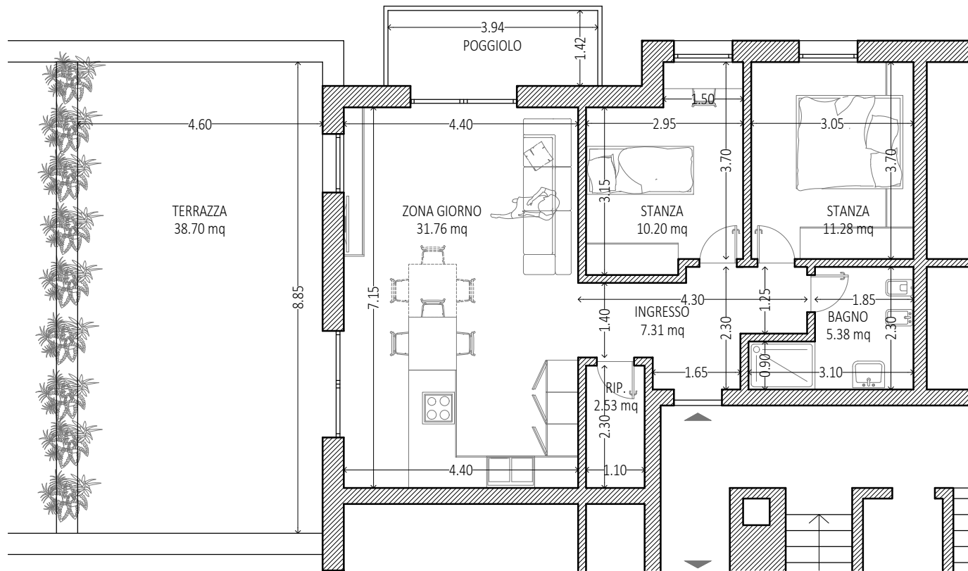
PIANTA APPARTAMENTO TERRAZZA _ secondo piano scala 1:100
